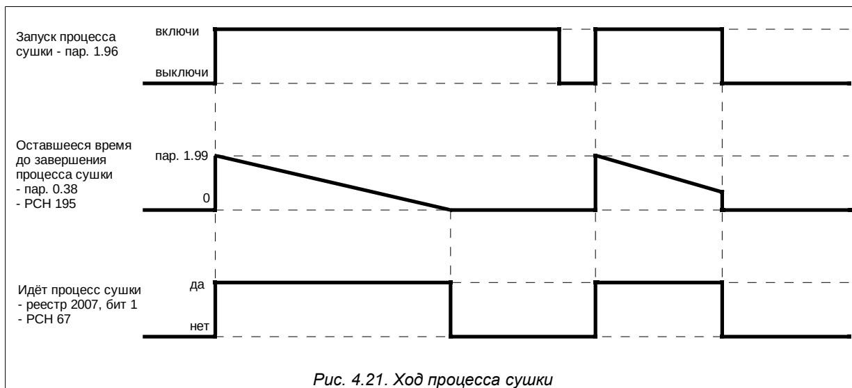
Рис. 4.21. Ход процесса сушки
